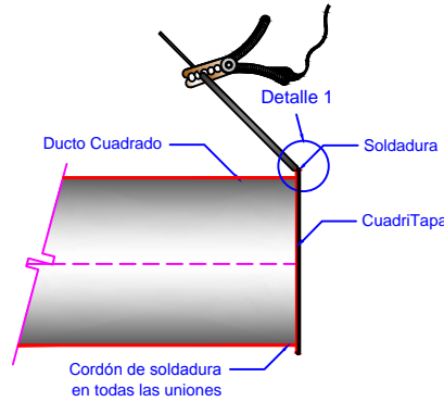
2. Montaje Lateral
