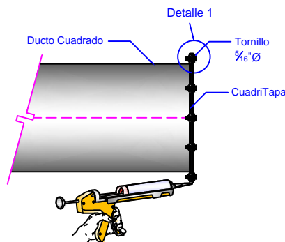
2. Montaje Lateral
